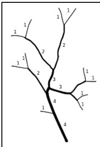
شکل ۱- نگاره شماتیک رتبه‌بندی رودخانه‌ها به روش استرالر [۷]
